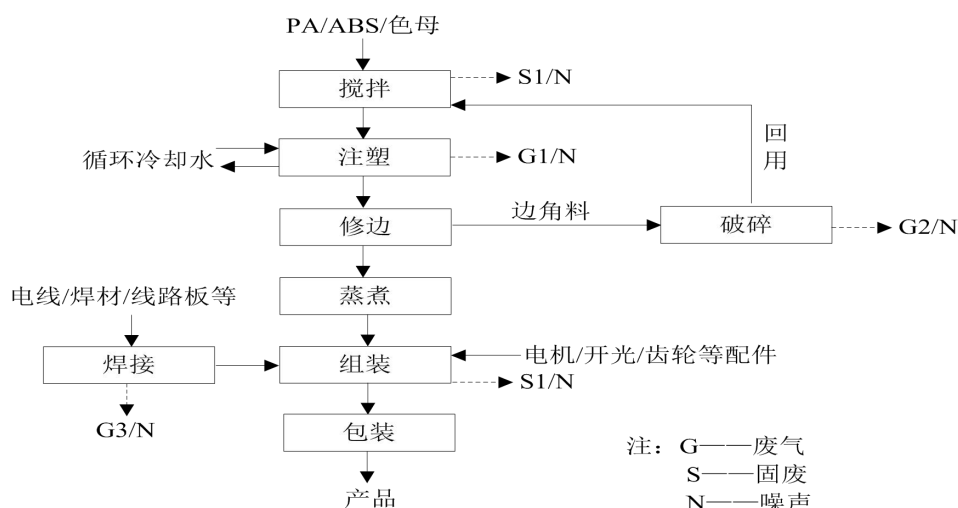
工艺流程图
