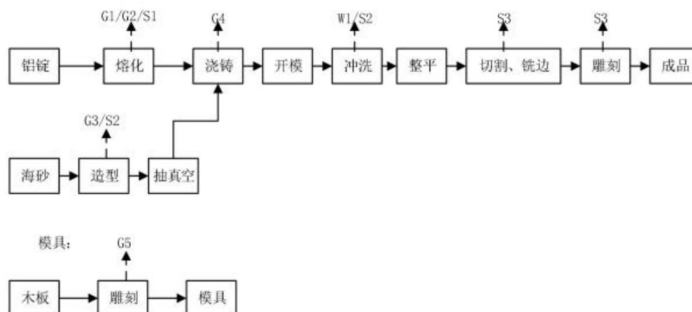
铸铝门面生产工艺流程图
